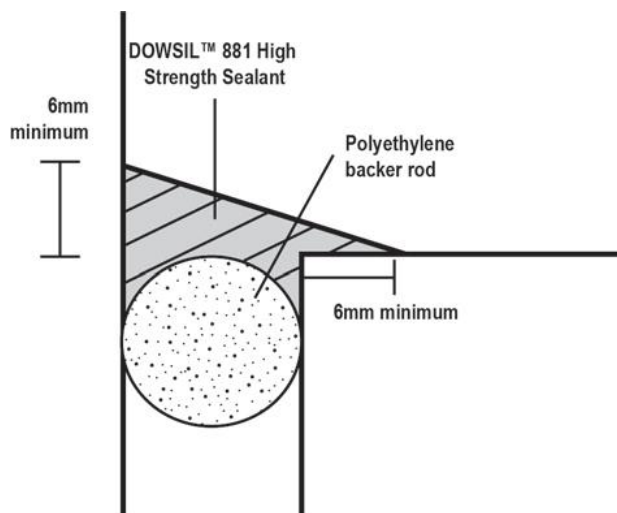
Obr. 3: Koutový spoj
