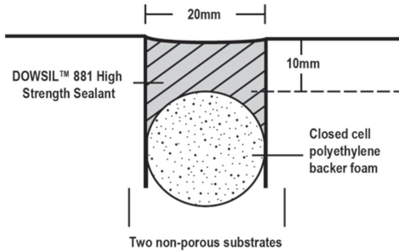
Obr. 2: Mělký spoj
