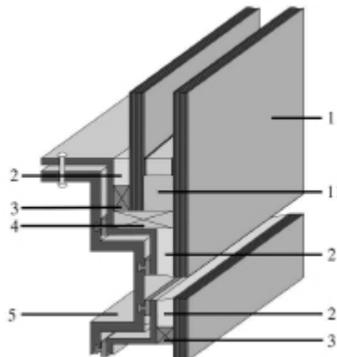
Obr. 5: Řešení se stupňovitým izolačním sklem.
