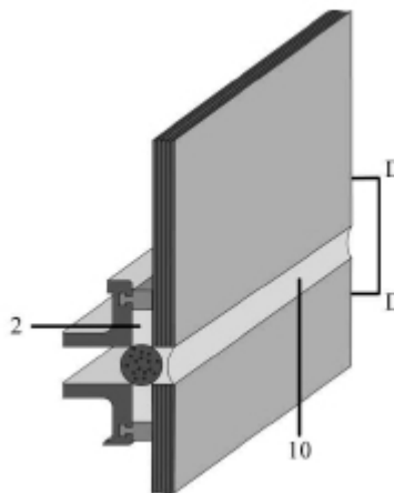
Obr. 5: Řešení se stupňovitým izolačním sklem.
